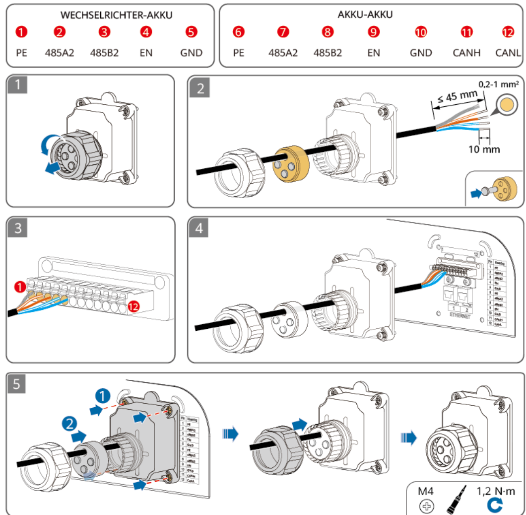
Afbeelding5-6 Signaalpoortaansluitingen
